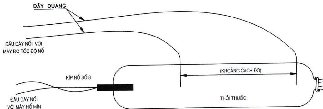
Hình 1 - Sơ đồ chuẩn bị mẫu và cách đầu dây với mẫu thuốc nổ
